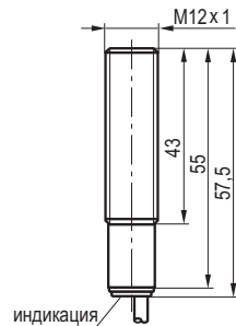
Габаритный чертеж
